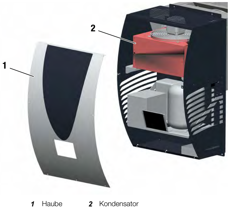
Fig. 17: Reinigung der Bauteile außen
