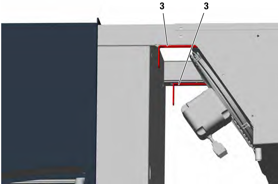
Fig. 9: Installation, Befestigung des eingehangen Geräts
